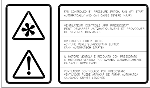
Şekil 4. Fan Uyarısı
