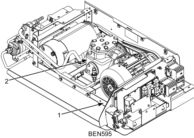
Şekil 12. Kondenser ve Bekleme Kompresörü Seri Numarası Konumları
